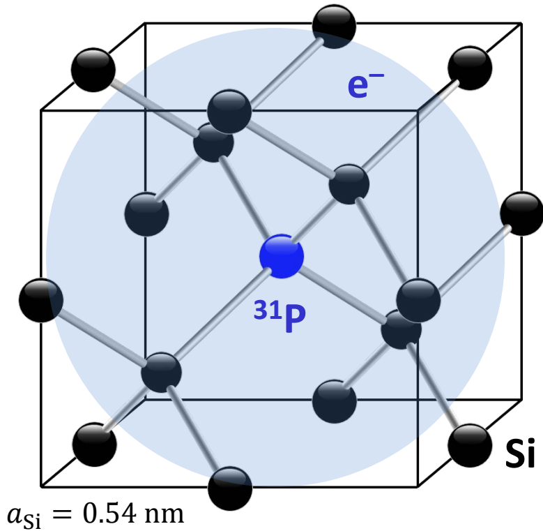
浅い不純物
